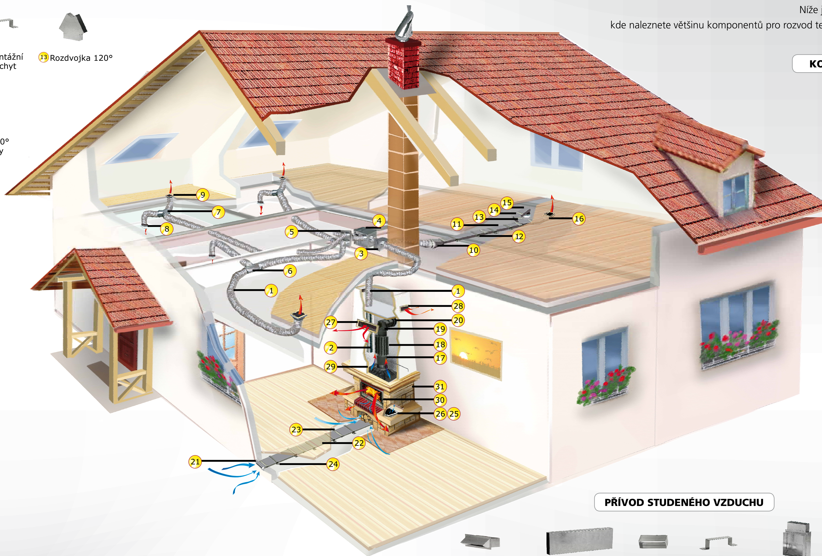
18 Trubka žebrovaná BERTRAMS
