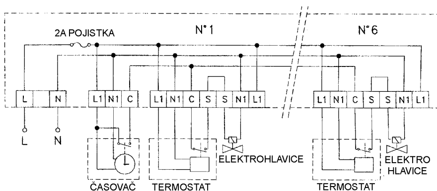
Obr.1: 88P3080653 vnitřní elektrické schéma zapojení
