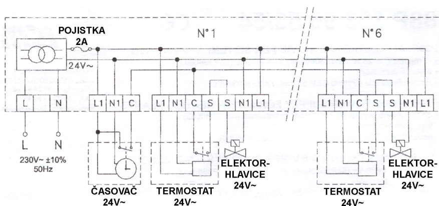
Obr.1: 88P3080653 vnitřní elektrické schéma zapojení
